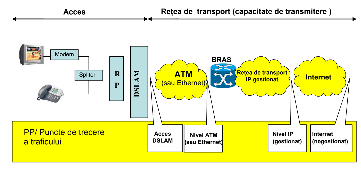
Figura 1: Acces cu ridicata în bandă largă (acces de tip „bit-stream” la bucla locală)
